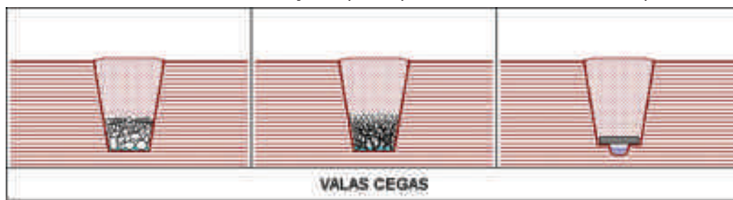
Figura 33 - Sistema de drenagem subterrânea por valas cegas
